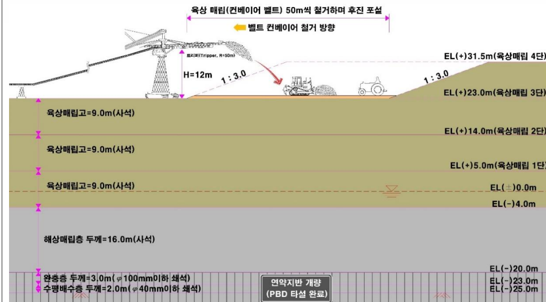
STEP 4 (4차 육상매립 EL+31.5)
