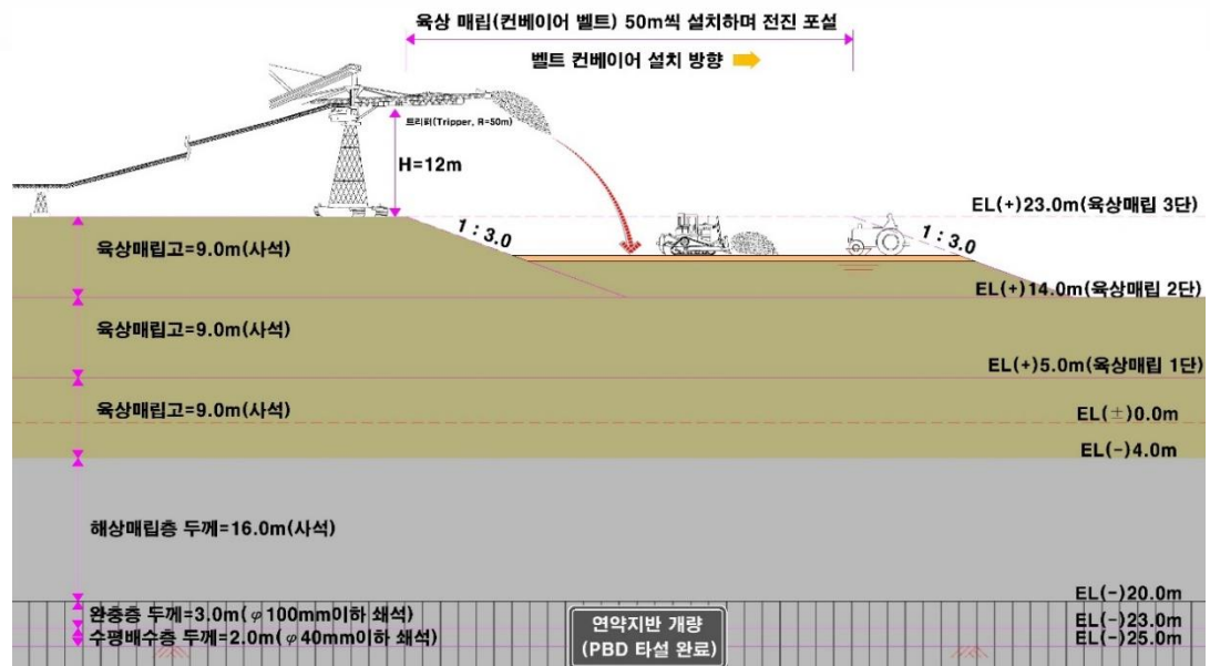
STEP 3 (3차 육상매립 EL+23.0)
